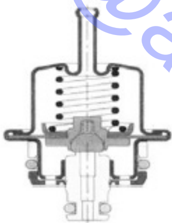
شکل ۳.۵۵ مقطع عرضی تنظیم کننده فشار سوخت
