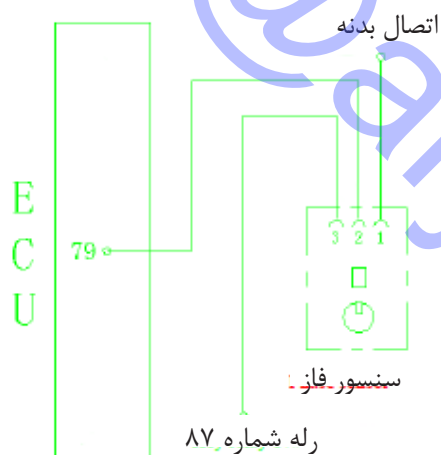
شکل ۳.۳۲ دیاگرام مدار سنسور فاز
