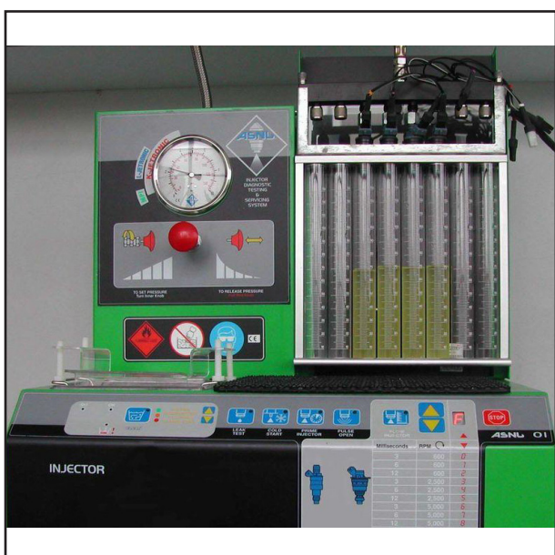
نام ابزار: دستگاه شست و شو و آنالیز انژکتور (نازل پاشش سوخت) کاربرد: شست و شو و تحلیل عملکرد انژکتورهای سوخت
